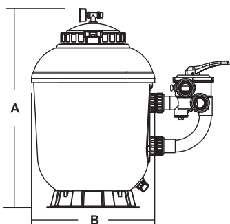
ABMESSUNGEN
